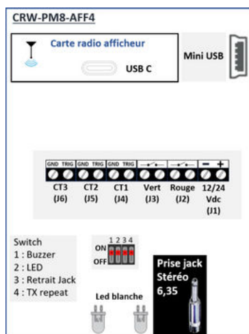
Bornier de raccordement débrochable à vis.
