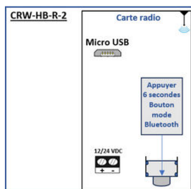
Bornier de raccordement débrochable à vis.
